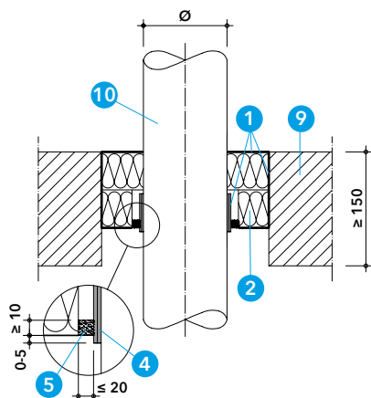
Detail T - prostup plastového potrubí bez izolace ve střezech 2)
