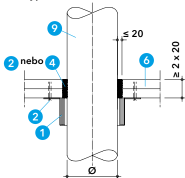
Detail V - průstup plastového potrubí v zavěšeném pohledu s manžetou PROMASTOP®-FC
