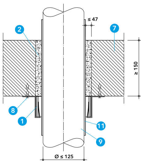
Detail D - průřez plastového potrubí do průměru 125 mm stropem
