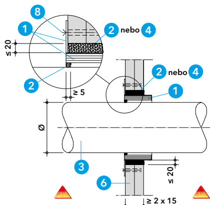
Detail U - průstup plastového potrubí v šachtové přičce s manžetou PROMASTOP®-FC - typ řešení č. 3
