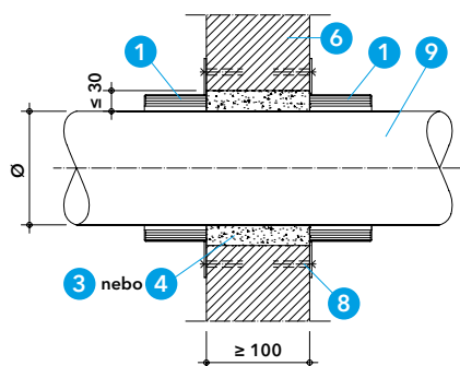
Detail E - průstup plastového potrubí v masivní stěně s manžetami PROMASTOP®-FC a maltou PROMASTOP®-M, popř. tmelem Promat® Ready Mix PRO
