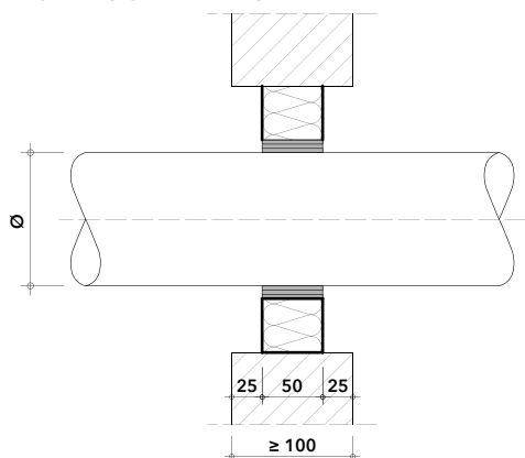
Detail T - prostup plastového potrubí bez izolace ve střezech 2)
