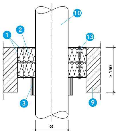
Detail N - průstup plastového potrubí ve stropěch 2) - přisazená varianta
