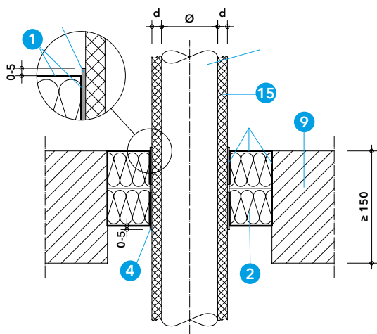
Detail Z - prostup vícevrstevných plastových potrubí s hliníkovým jádrem ve stropě 2)
