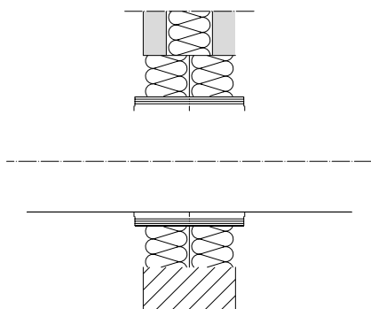
Detail N - průstup plastového potrubí ve stropěch 2) - přisazená varianta
