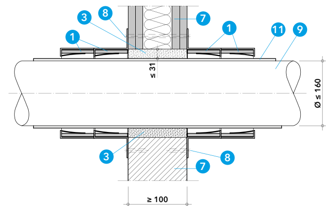
Detail C - průřez plastového potrubí do průměru 160 mm stěnou
