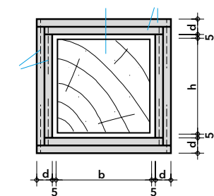
Příčný řez
