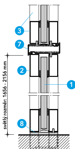
Detail B - svislý řez A-A
