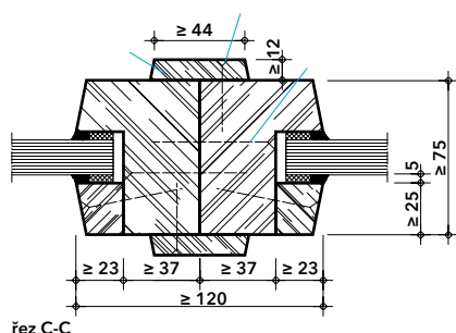
Detail D - spojení dvou rámců
