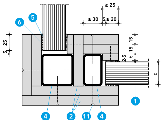
Detail D - posuvné připojení k masivnímu stropu
