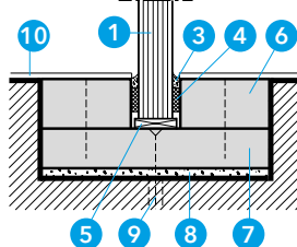
Detail C - nosná konzole
