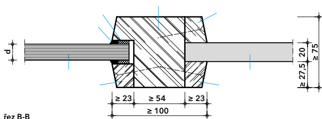
Detail H - plná výplň PROMATECT®-H (≤ EI 30/EW 45)
