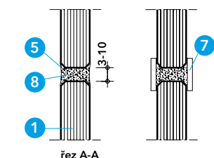
Detail C - spáry mezi skly
