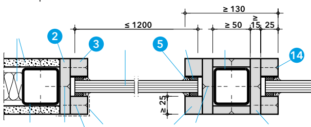
řez A-A
