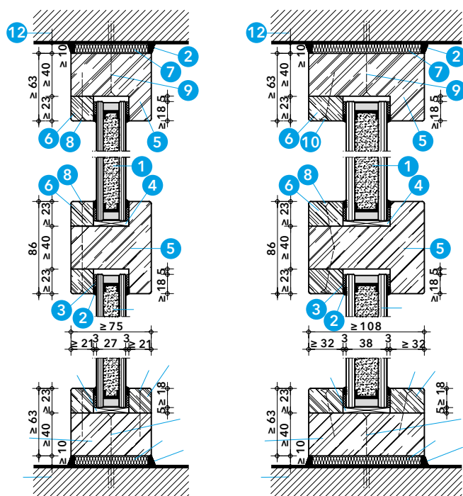
řez B-B (El 30)
