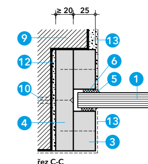
Detail E - připojení ke stěně
