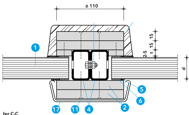
Detail C - zakrytí, vazební profil
