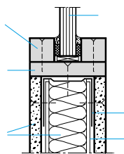
řez D-D
