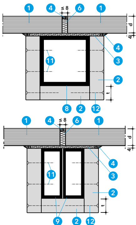
Detail B - středový profil (alternativy)
