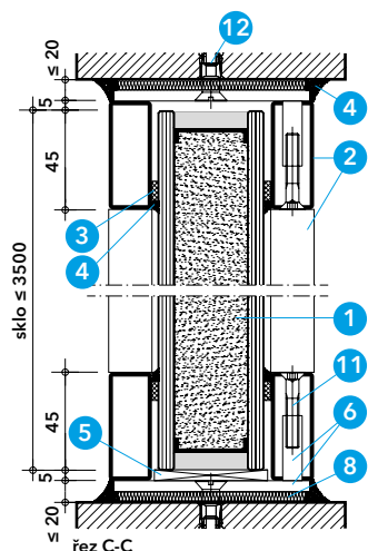
Detail C - svislý řez
